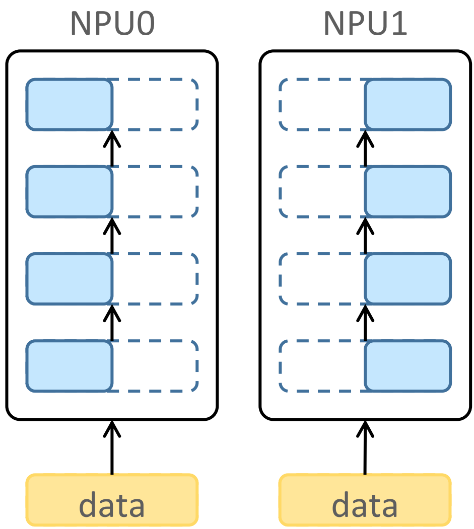
张量并行 tensor parallel
