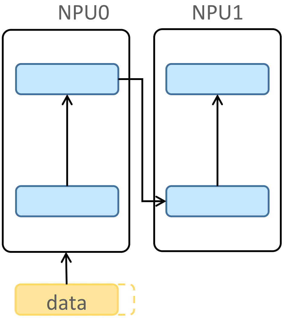
流水线并行 pipeline parallel
