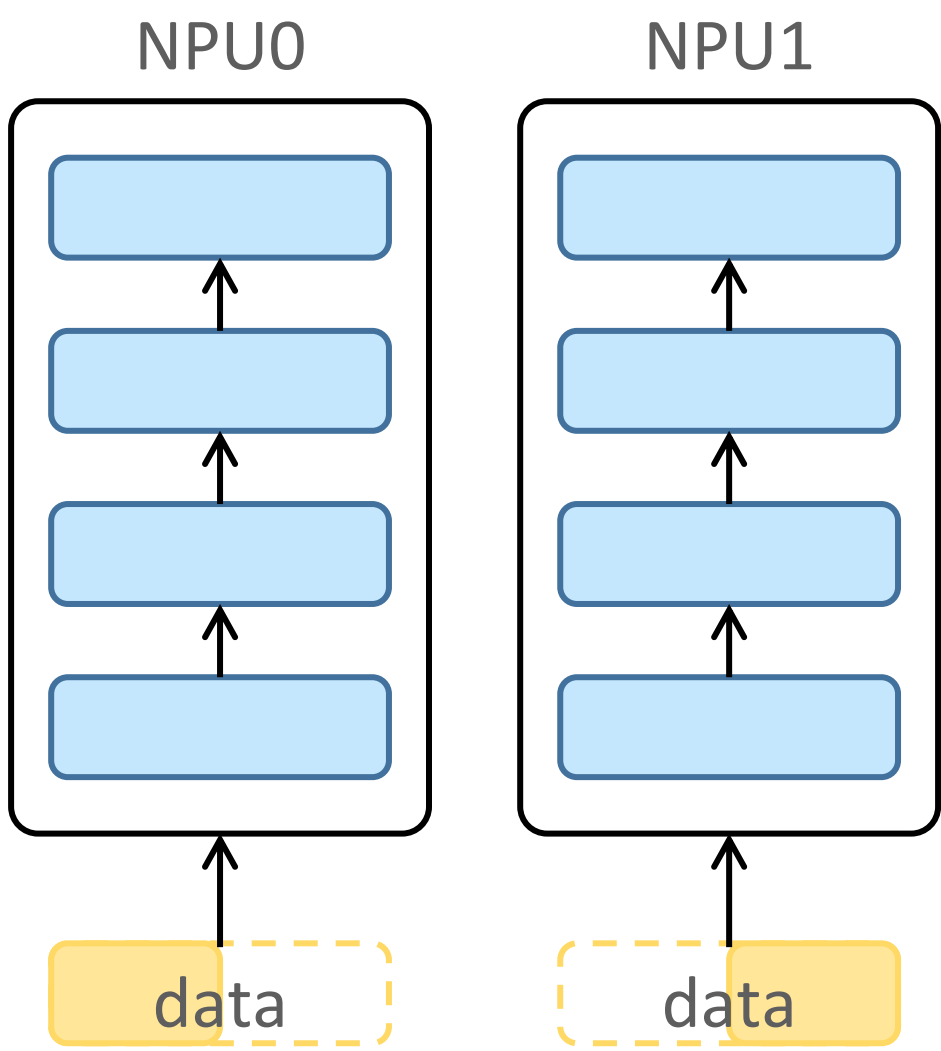
数据并行 data parallel
